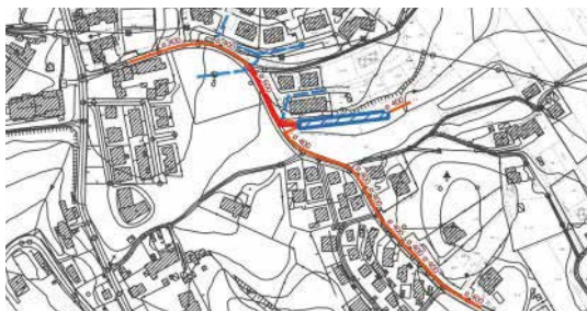
Inquadramento delle opere in progetto su Carta Tecnica Regionale. In blu tratteggiato sono riportati i tratti di fognatura bianca già esistenti, in rosso le condotte di progetto e il poligono blu indica l'area dove è previsto l'invaso.
